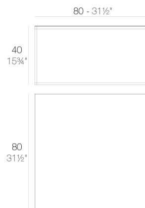
SUAVE Mesa Baja 80x80x40 SUAVE Low Table 31½x31½x15¾
